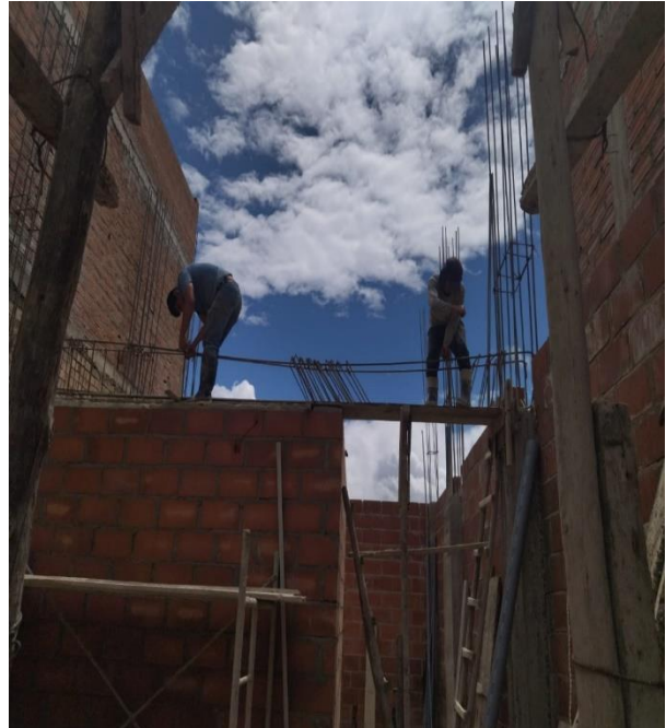
Fotografía 26. Acero en vigas V-05
