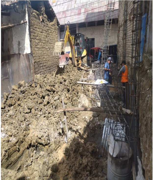
Fotografía 42. Habilitación de acero en columnas V-09
