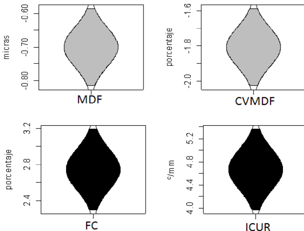
Figura 1. Intervalos de confianza (alfa=0.05) de los cambios de cuatro características tecnológicas de la fibra de llama Chaku por efecto del descerदार (MDF = Media de diámetro de fibra, CVMDF = Coeficiente de variación de la MDF, F = Factor de confort, ICU = Índice de curvatura)
